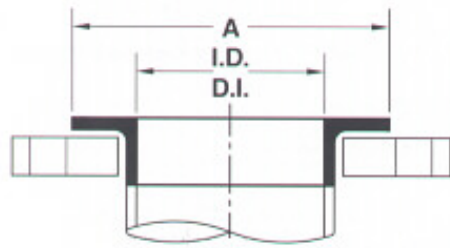
BUTT WELD / BOUT À SOUDER
